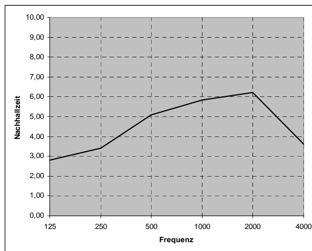
Abbildung 3: Prognostizierte Nachhallzeit ohne akustische Maßnahmen, ohne Besucher
