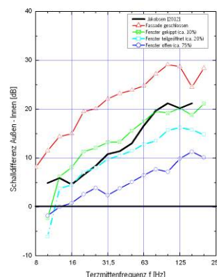
Abbildung 3: Gemitteltes Übertragungsmaß \Delta L = \text{Außenpegel} - \text{Innenpegel} im konventionellen Wohnungsbau bei (teil-)geöffnetem Fenster
